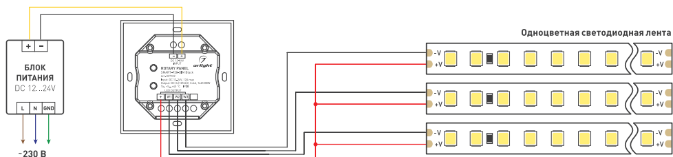
Рис. 1. Подключение одноцветной светодиодной ленты
